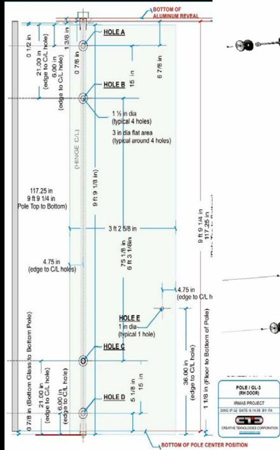
Pole Hinge
